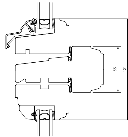
Vertikalsnitt 2-luft Vertical section 2-lights
